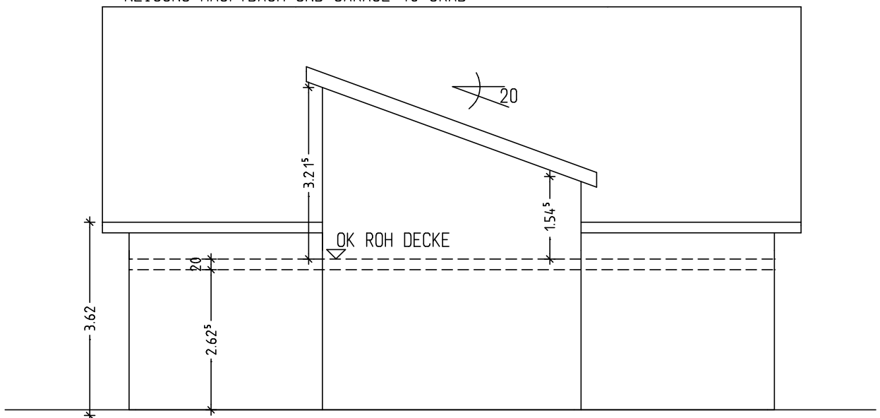
NEIGUNG HAUPTDACH UND GARAGE 40 GRAD
